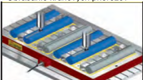
Obrábanie viacerých kusov
