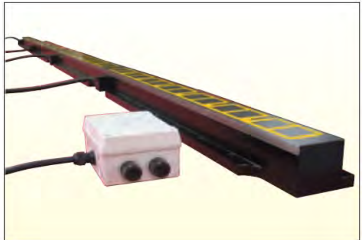
EEPM platňa použitá na 5 osom obrábacom CNC centre
